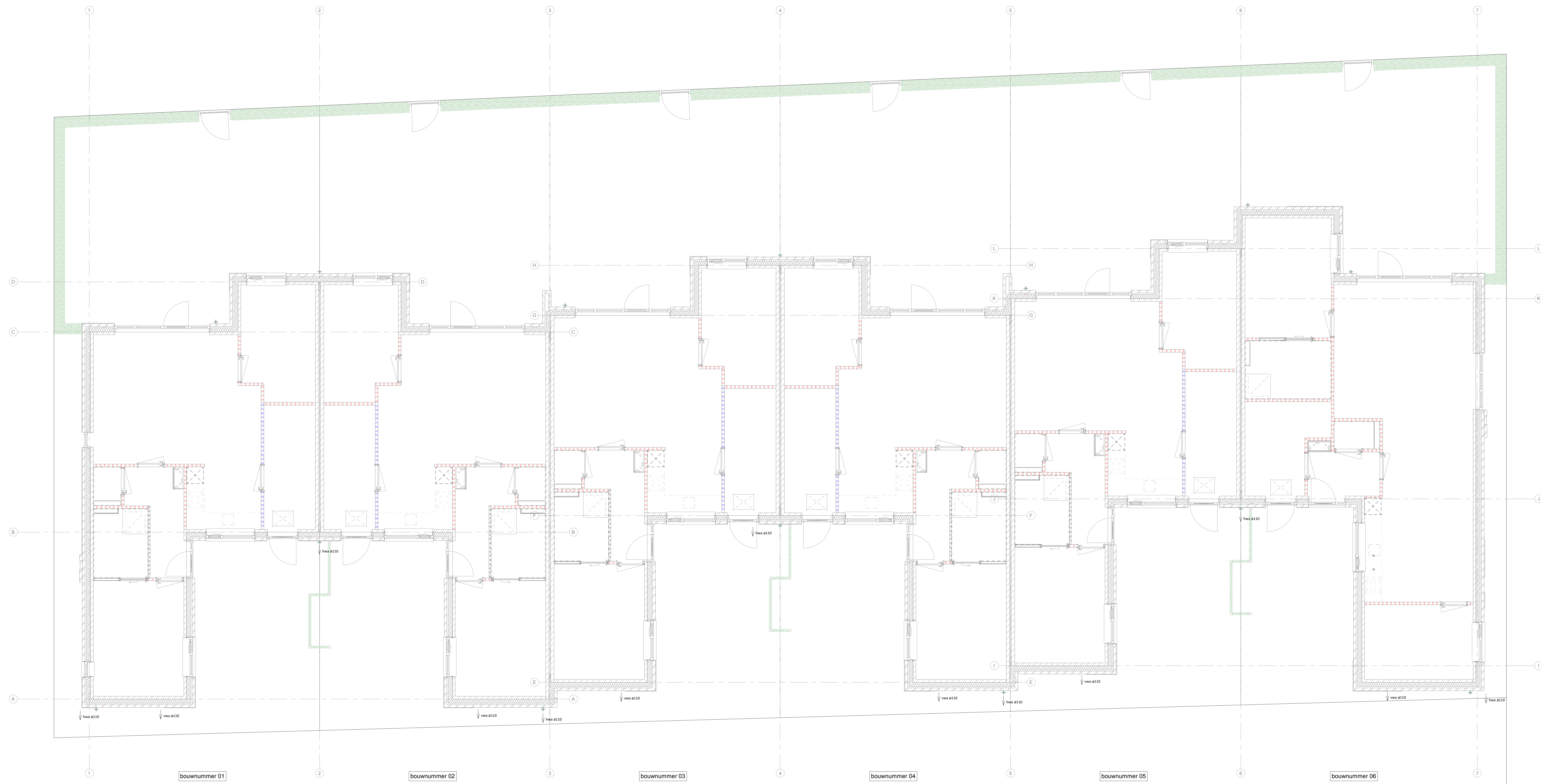
begane grond 01-06 HWA + VWA
